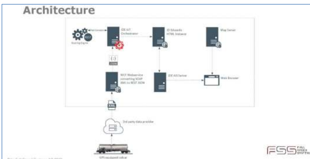
Abbildung 6; Architektur der Lösung inkl. JDE IoT Orchestrator
